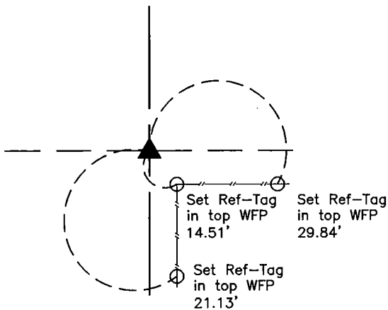
SE Corner NW 1/4-SW 1/4 Set 1/2"Ø Rebar w/ Orange Plastic Cap PLS 17939
