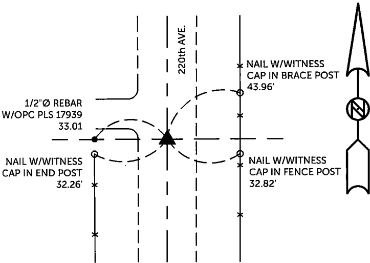
SE CORNER NE 1/4 - SE 1/4 SET 1/2" REBAR W/ORANGE CAP #17939
